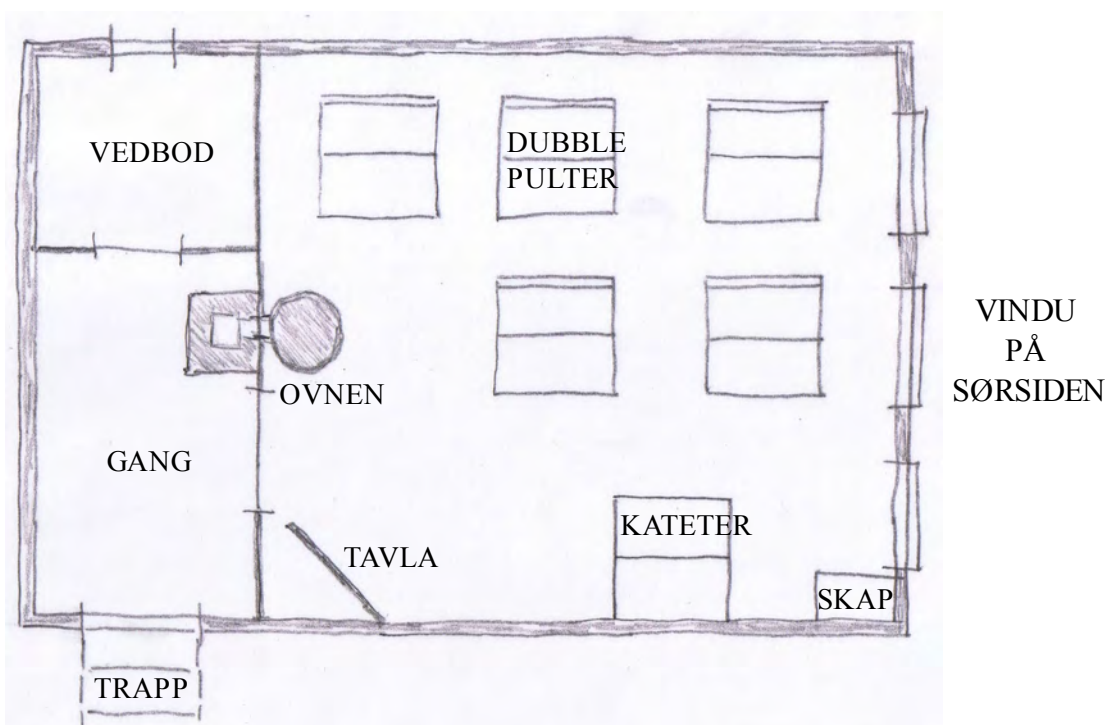
Skulen var 7,5 meter lang og 6 meter breid. Tegningen viser hvordan det var innvendig slik Solveig husker det. Tegning: Paul Tengedal 2012.
