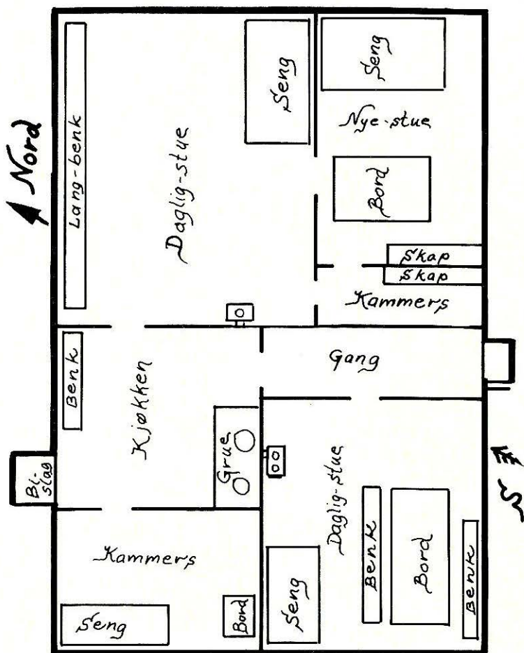
Grunnriss av Tybringhuset, 1. etasje
